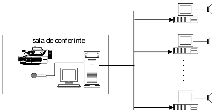
(a) Distributia audio-video locala pe LAN Ethernet.
